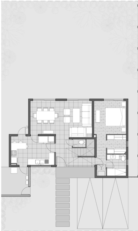
Piso 1
