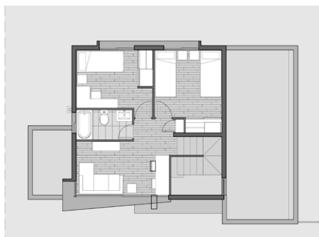
Piso 2
