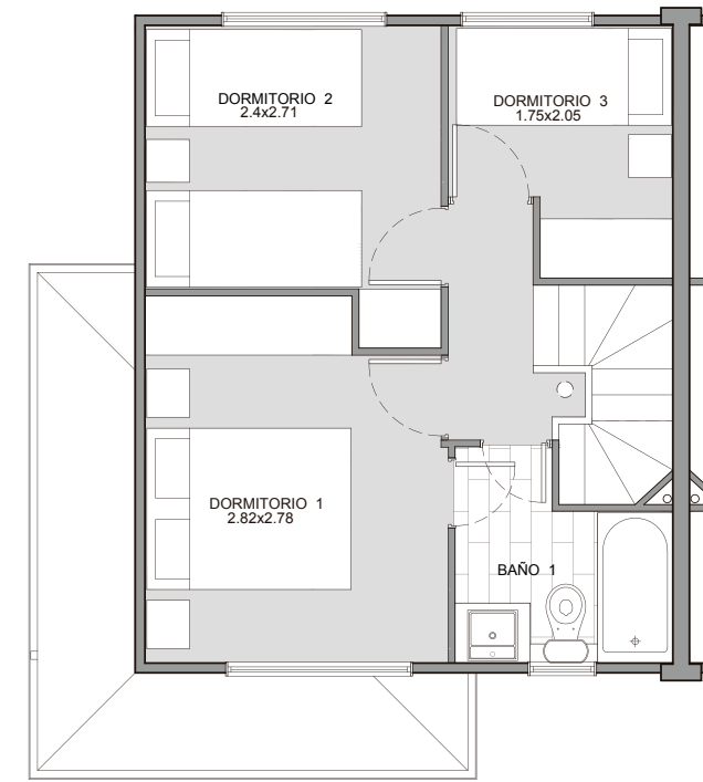
Planta Base Nivel 2
