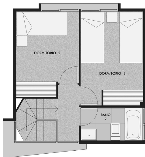
PLANTA 2° PISO
